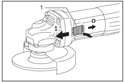
► 1. Slide switch
